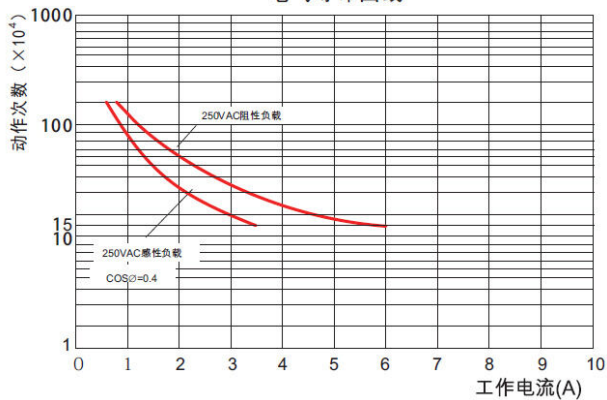
电气寿命曲线
